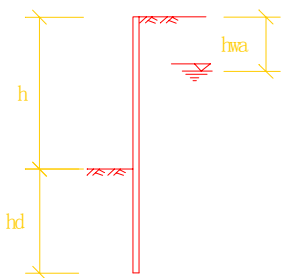
图 4.1.3 渗透稳定 计算简图
