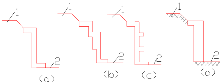
图 7.2.2 拱墙截面构造示意简图
