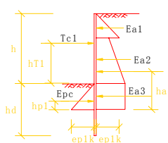
图 4.1.1-2 单层支点支护结构 支点力计算简图
