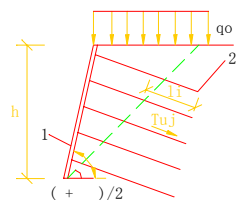
图 6.1.4 土钉抗拉承载力计算简图
