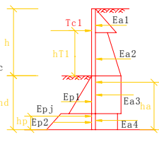
图 4.1.1-3 单层支点支护结构 嵌固深度计算简图
