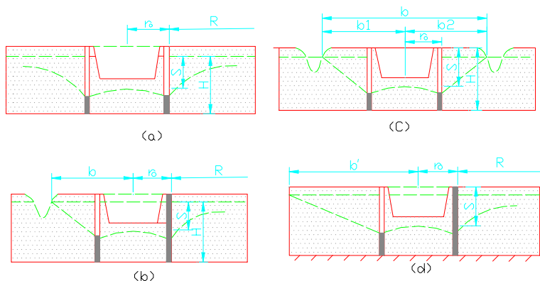
图 F. 0. 1 均质含水层潜水完整井基坑涌水量计算简图
