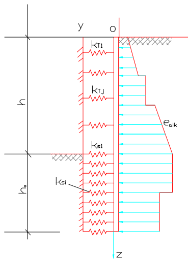
图 B. 0. 1 计算简图
