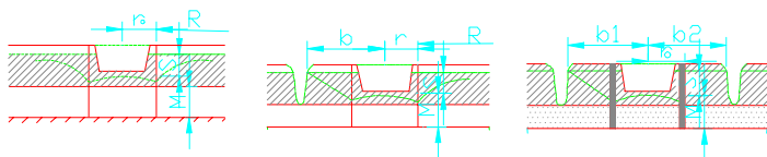
图 F. 0.3 均质含水层承压水完整井基坑涌水量计算图
