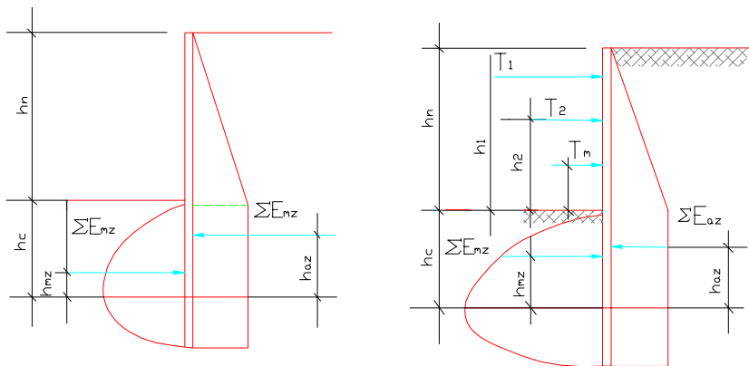
图 B. 0. 5 内力计算简图
