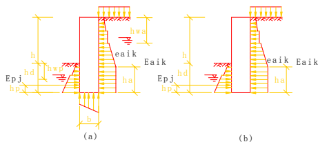
图 5.2.1 水泥土墙宽度计算简图
