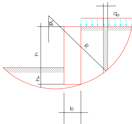
图 A. 0.1 嵌固深度计算简图
