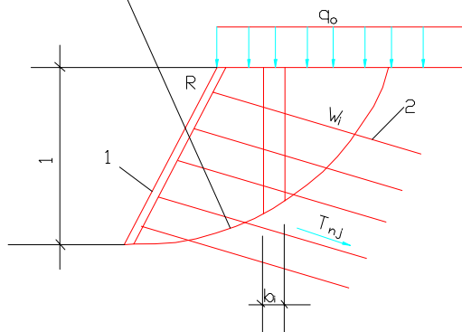
图 6.2.1 整体稳定性验算简图
