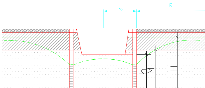
图 F.0.5 均质含水层承压~潜水非完整井基坑涌水量计算图
