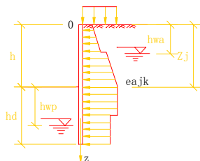
图 3.4.1 水平荷载标准值计算简图
