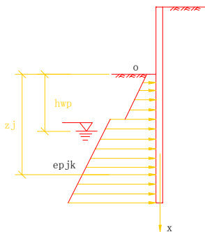
图 3.5.1 水平抗力标准值计算图
