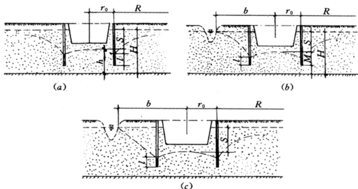
图 F. 0. 2 均质含水层潜水非完整井涌水量计算简图
