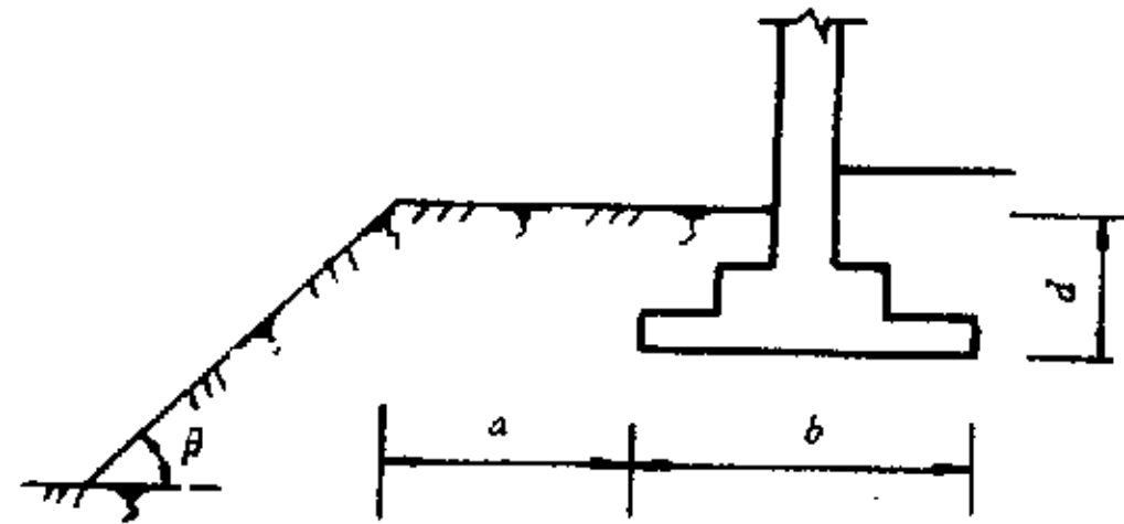
图 6.3.3 基础底面外边缘线至坡顶的水平距离示意图
