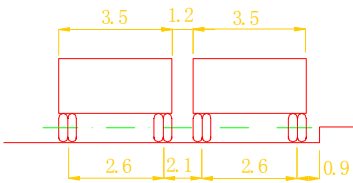
40t 汽车横向布置
