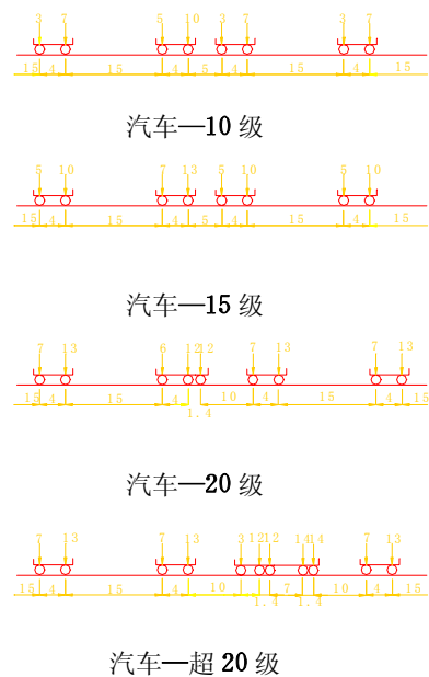
图 5.5.1—1 一般载重汽车车队纵向排列
