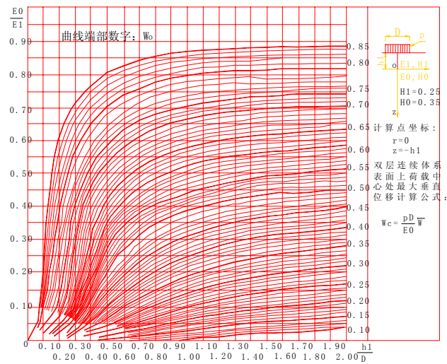
图 4.3.7 弹性层状体系精确解图解
