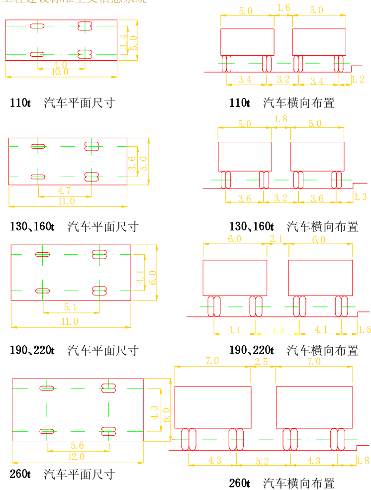
图 5.5.2—2 重型自卸汽车平面尺寸和横向布置
