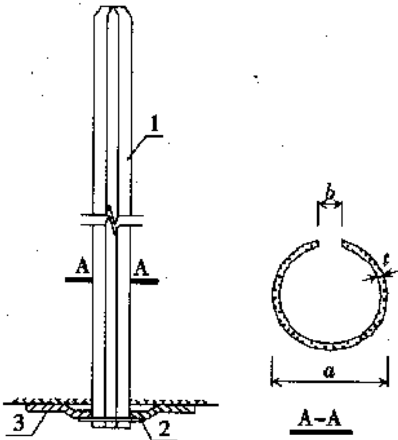
图 A.0.5 缝管锚杆
