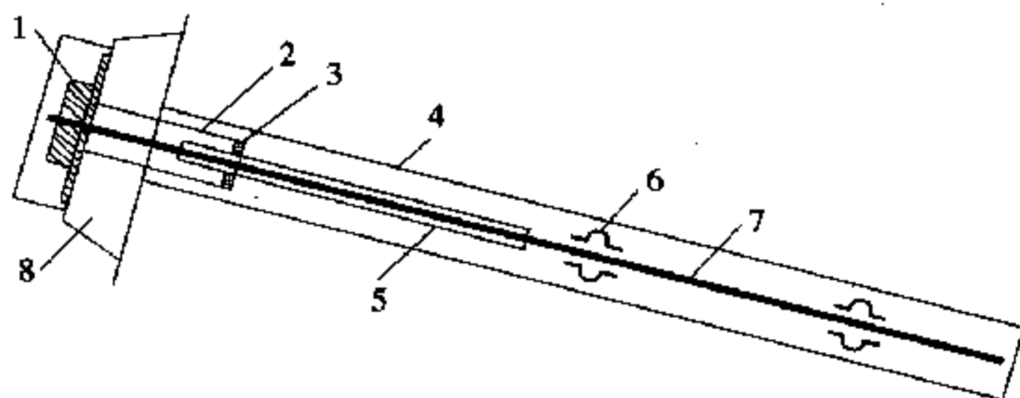
图 6.2.1-2 锚杆 II 级防护构造
